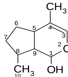
Иридоидаль (лактонная форма)
