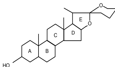
Стероидный сапонин спиростанового типа
