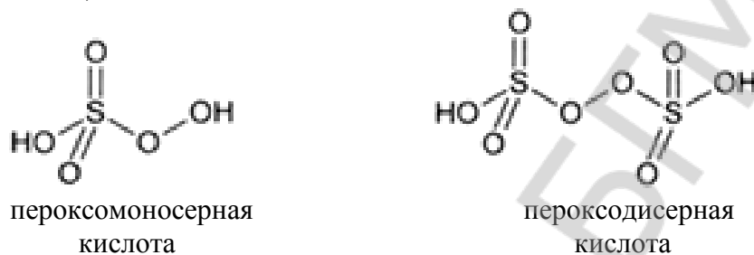
Рис. 14.5. Строение пероксокислот
