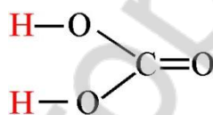
Рис. 12.4. Схема строения угольной кислоты
